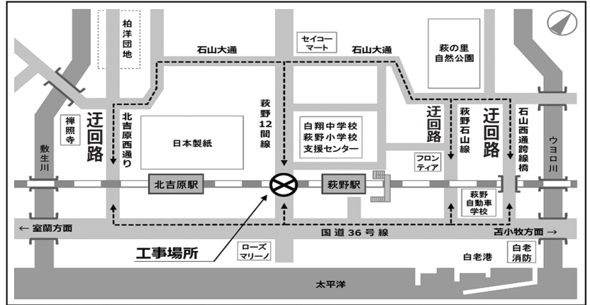
迂回路平面図
